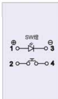
電路圖
