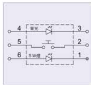
XPB電路圖
