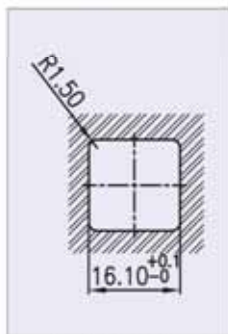
鍍金開孔尺寸
