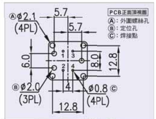
RHB3.RHB4腳位定義圖
