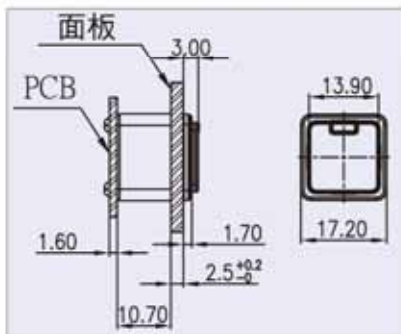
RHB3.RHB4尺寸圖
