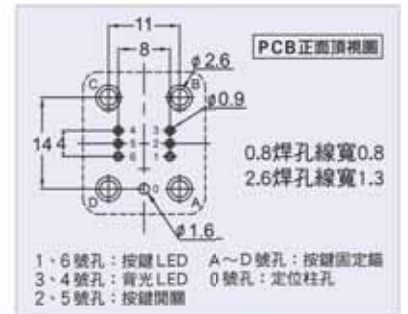
RHB1.RHB2腳位定義圖
