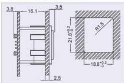
RHB1.RHB2鍍金開孔圖
